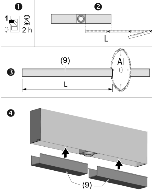
Bild 5: Profilabdeckung montieren
